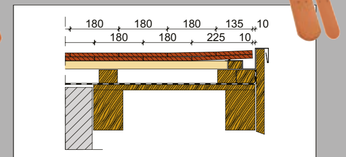
Oromszegély 3/4 és 5/4 hódfarkú cserepekkel
