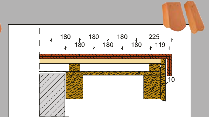
Oromszegély 3/4 és 5/4 szegélycserepekkel
