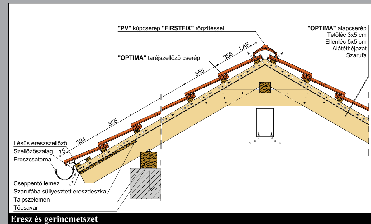
Eresz és gerincmetszet
