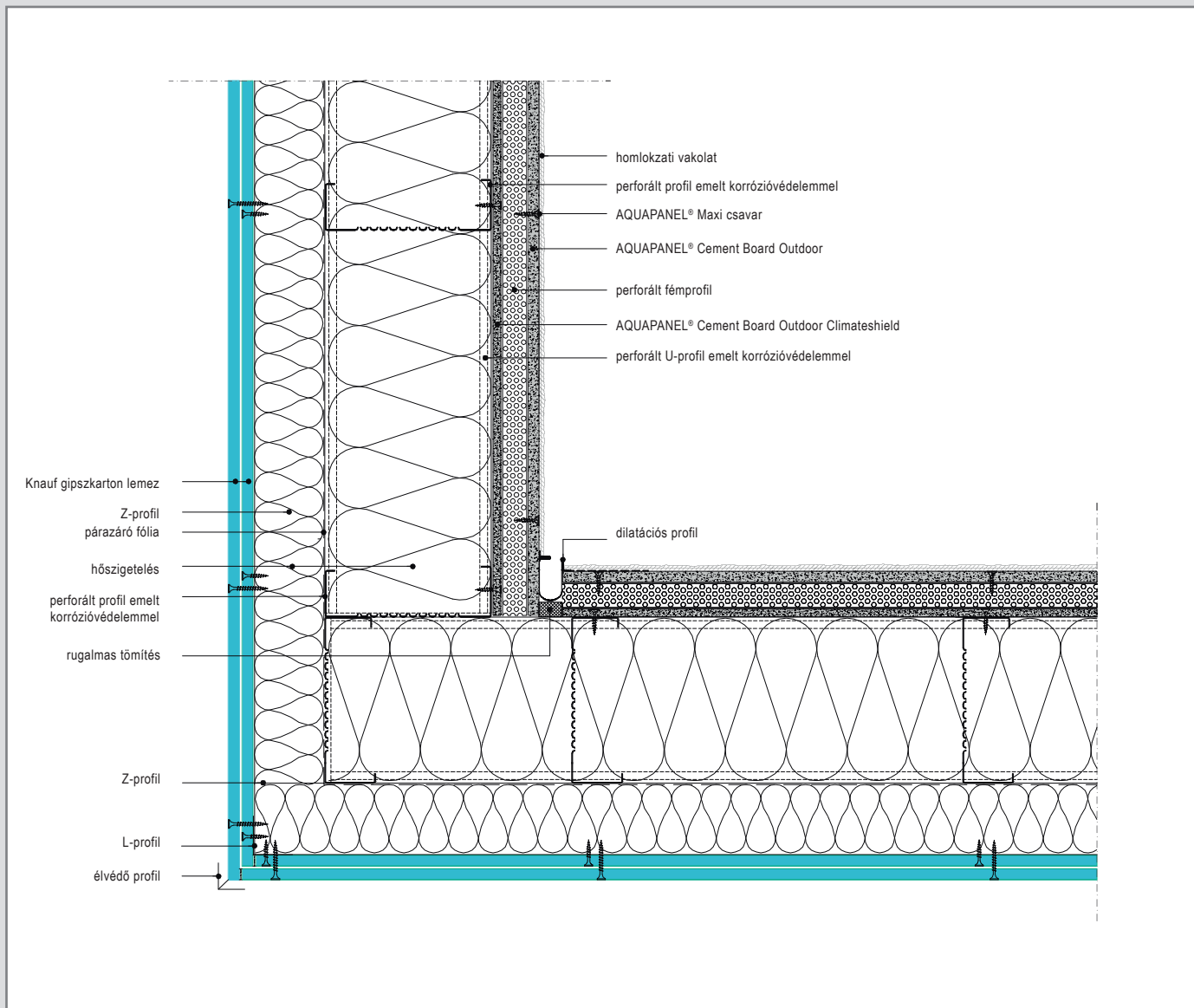
W684W-DBFU1 Kiszellőtetett negatív sarok mozgási hézaggal
