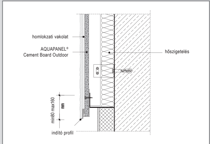
W684T-SO-V1 Lábazat kialakítás
