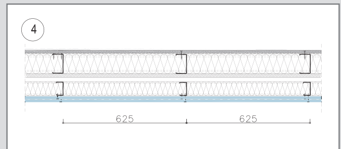
04. Kettős váz kettős hőszigeteléssel
