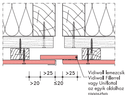
S1 Mozgási hézag tűzvédelmi kialakításban
