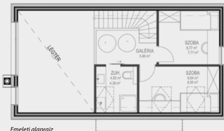
Emeleti alaprajz
