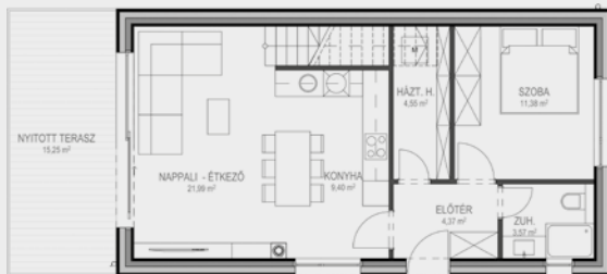
Földszint alaprajz
