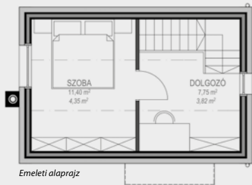
Emeleti alaprajz
