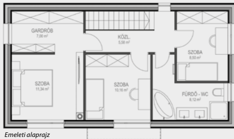
Emelet alaprajz
