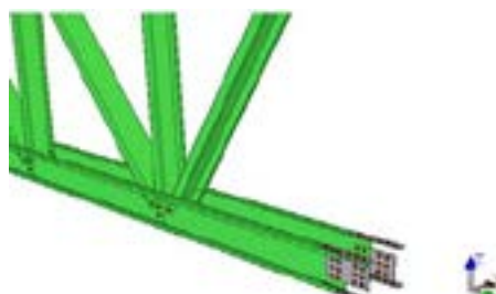
4. ábra. Felső és alsó övrúd helyszíni illesztése
