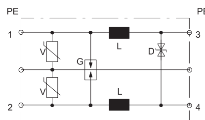
Kapcsolási rajz
