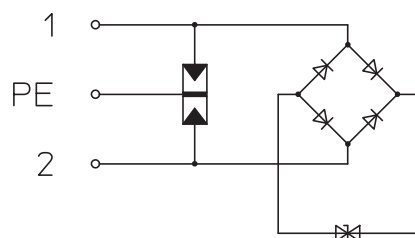
Kapcsolási rajz
