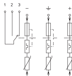
Kapcsolási rajz
