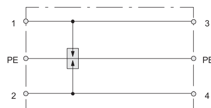
Kapcsolási rajz
