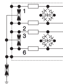
Kapcsolási rajz
