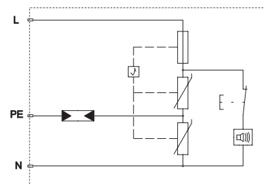
Kapcsolási rajz
